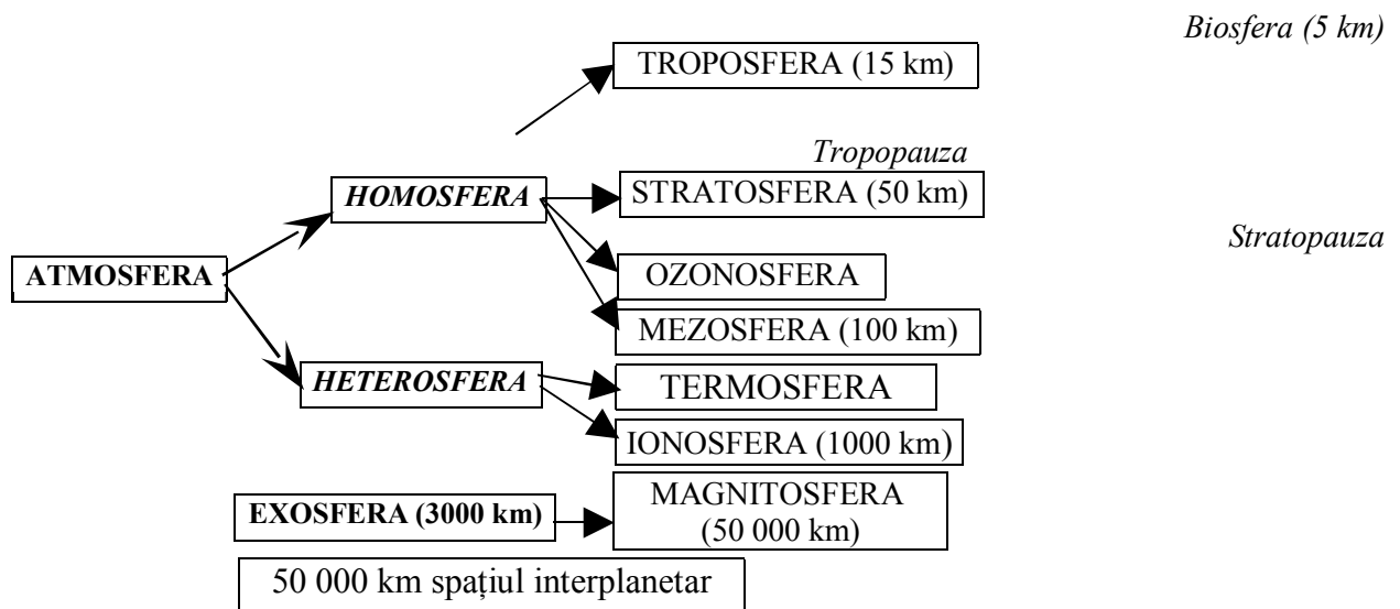
Fig. 6. Stratificarea atmosferei.
