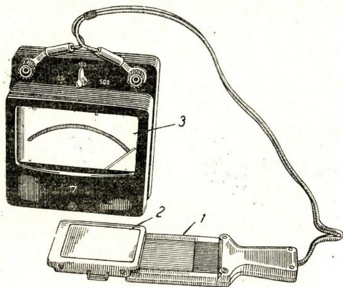
fig. 23. Luxmetru 1 — fotoelement; 2 — filtru; 3 — galvanometru
