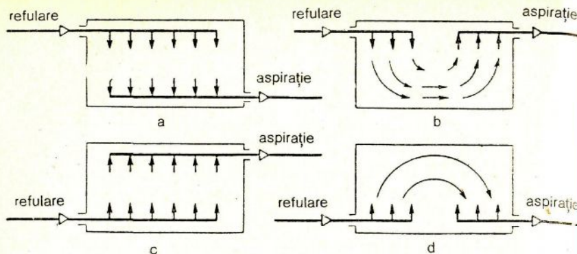
fig. 18. Schema refulării și aspirației aerului în încăperi a - de sus în jos; b - de sus în sus; c - de jos în sus; d - de jos în jos
