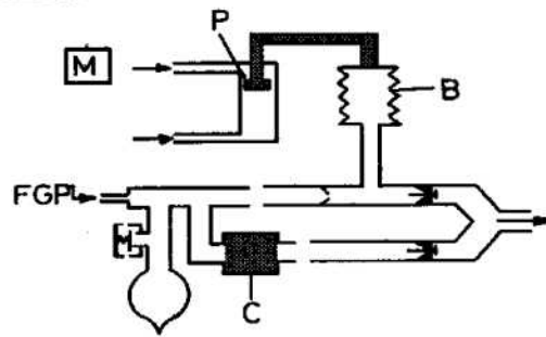
Fig.17.6 Schema ventilator cu burduf și piston. M=motor, P=piston, B=burduf, FGP=flux gaze proaspete, C=canistra calce sodată.
