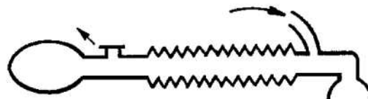
Fig.16.13 Schemă SRA Mapleson D.
