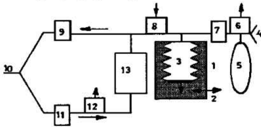
Fig.17.12 Dispozitiv "bellow in bottle" descendent. 1=container rigid, 2=gaz motor, 3=burduf de insuflare cu greutate, 4=FGP, 5=rezervor pentru FGP în insuflare, 6=supapă evacuare reglată manual, 7=supapă izolare balon reglată de ventilator, 8=supapă admisie aer ambient (se deschide dacă presiunea este negativă în sistem), 9=valvă inspiratorie, 10=racord pacient, 11=valvă expiratorie, 12=supapă evacuare comandată de ventilator, 13=canistră calce sodată.
