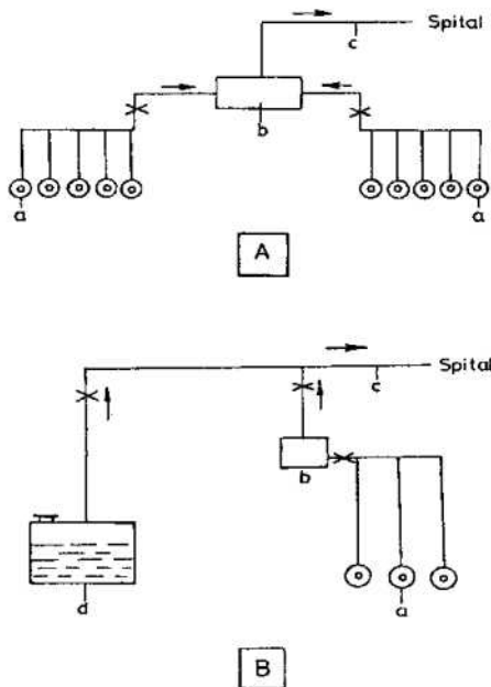
Fig.15.5 Schema stației centrale de gaze. A-cu butelii, a-baterii de rezervă, b-sistem de conectare automată a sau d, c-sistem de distribuție. B-cu gaze lichefiate, d-tanc pentru gaze lichefiate și evaporare, a-baterii de rezervă, b-sistem de conectare automată a sau d, c-sistem de distribuție.
