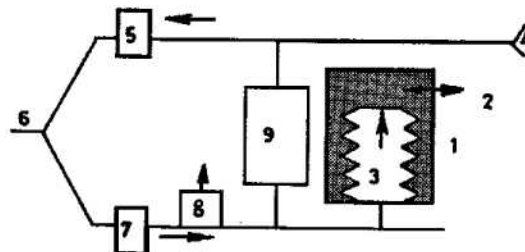
Fig.17.11 Dispozitiv "bellow in bottle" ascendent. 1=container rigid, 2=gaz motor, 3=burduf de insuflare, 4=FGP, 5=valvă inspiratorie, 6=racord pacient, 7=valvă expiratorie, 8=supapă evacuare comandată de ventilator, 9=canistră calce sodată.
