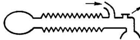
Fig.16.11 Schemă SRA Mapleson B.
