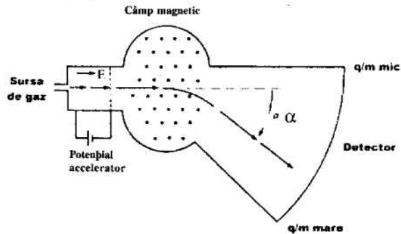
Fig.22.6 Principiul funcționării spectrometrului de masă (după Vender GS și Gilbert HC, 1997).
