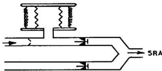
Fig.17.5 Ventilator cu burduf prevăzută cu arc.
