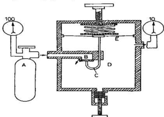
Fig. 15.7 Schema unui reductor cu o treaptă. A-butelie, B-camera de presiune înaltă, C-tija cu sertar obturator, D-camera de presiune joasă, E-membrana cu excursii limitate de arc.
