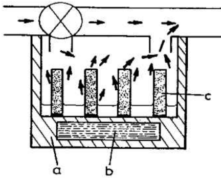
Fig. 15.15 Ilustrarea principiului termostatic. a-cuva de cupru, b-manșon de apă, c-bronz sinterizat.
