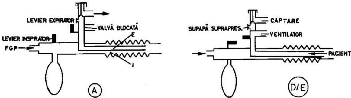
Fig.16.18 Schemă SRA ADE Humphrey.
