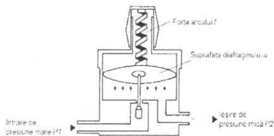
Fig.1.2 Valva reductoare de presiune.
