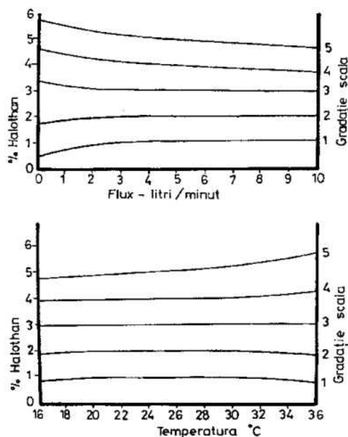
Fig.15.14 Ilustrarea curbelor de vaporizare în funcție de temperatură și flux de gaz (vaporizor Sigma-Penlon).
