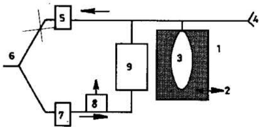
Fig.17.10 Dispozitiv "bag in bottle". 1=container rigid, 2=gaz motor, 3=balon de insuflare (FGP+gaz expirat), 4=FGP, 5=valvă inspiratorie, 6=racord pacient, 7=valvă expiratorie, 8=supapă evacuare (închisă în inspirație-deschisă în expirație), 9=canistră calce sodată.
