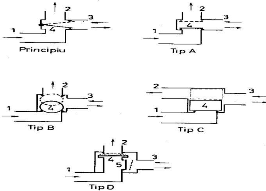
Fig.16.20 Valva unidirecțională negravitațională.
