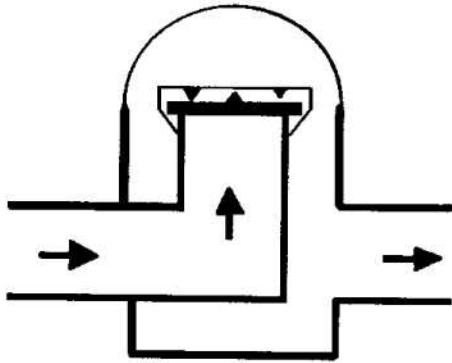
Fig.16.19 Valva unidirecțională gravitațională.
