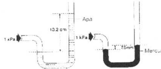
Fig.1.4 Manometrul cu apă și manometrul cu mercur.
