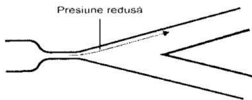
Fig.1.13 Efectul Coandă.
