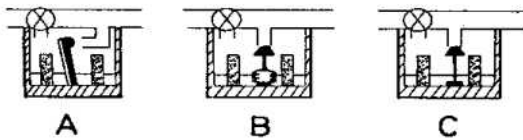
Fig. 15.16 Ilustrarea principiului termocompensării. A-lama bimetalică, B-burdof, C-tijă metalică.
