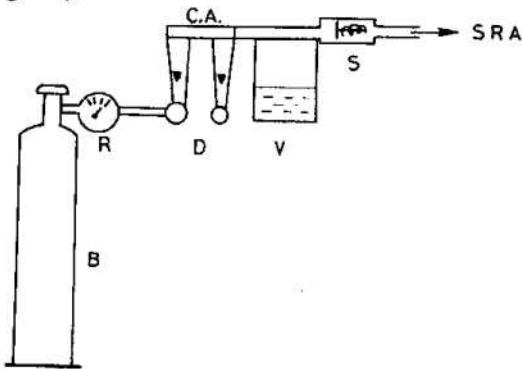
Fig.15.1 Schema mașinii de gaze. B-butelia, R-reductor, D-debitmetre, CA-camera amestec, V-vaporizor, S-supapă unidirecțională, SRA-sistem respirator anestezic.
