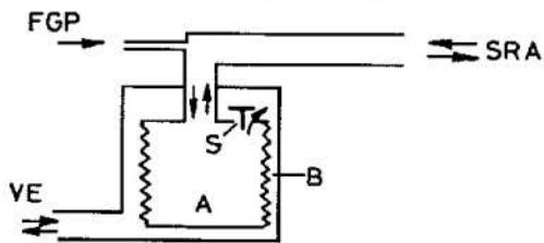
Fig.17.9 Schema unui dispozitiv cu circuit primar și secundar. A=burduf-circuit primar, S=supapă suprapresiune, FGP=flux gaze proaspete, SRA=sistem respirator anestezic, B=container rigid-circuit secundar, VE=gaz motor de la ventilator.
