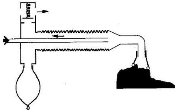
Fig.16.14 Schemă SRA Bain.
