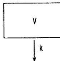
Fig.8.9 Modelul unicompartimental.
