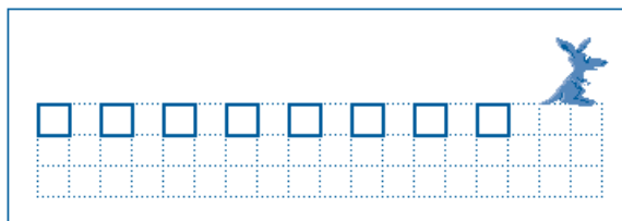
Рис. 5.3. Рисование квадратов
