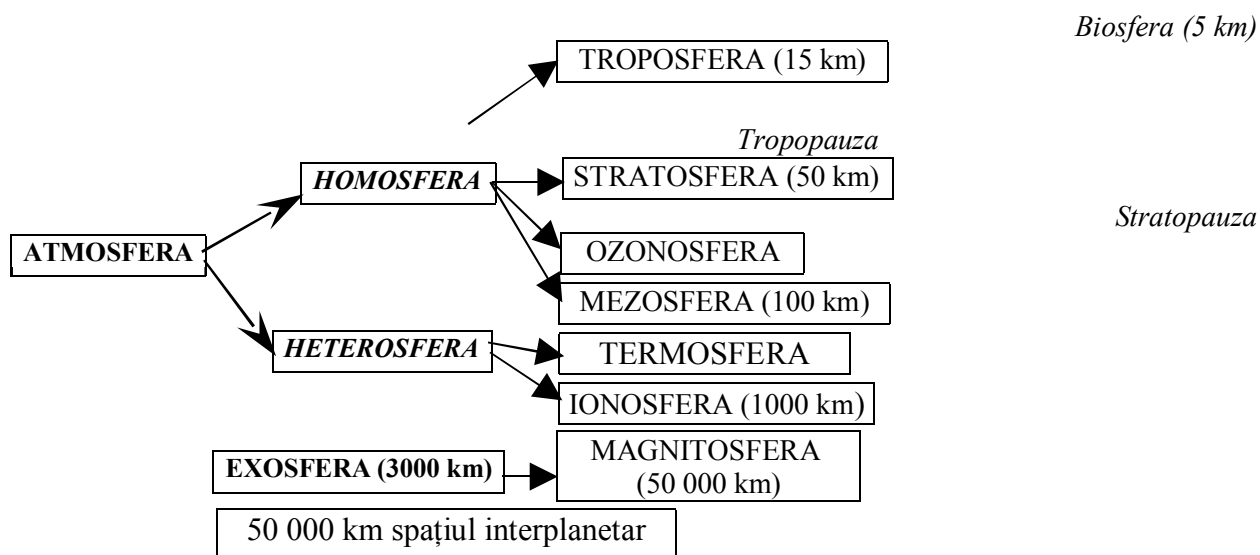
Fig. 6. Stratificarea atmosferei.
