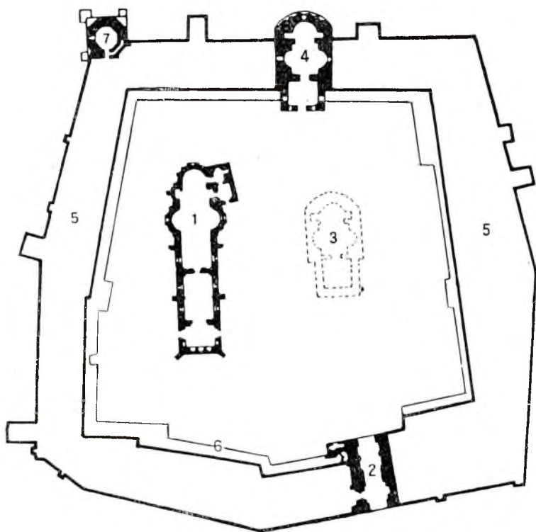
Mănăstirea Neamț plan.
