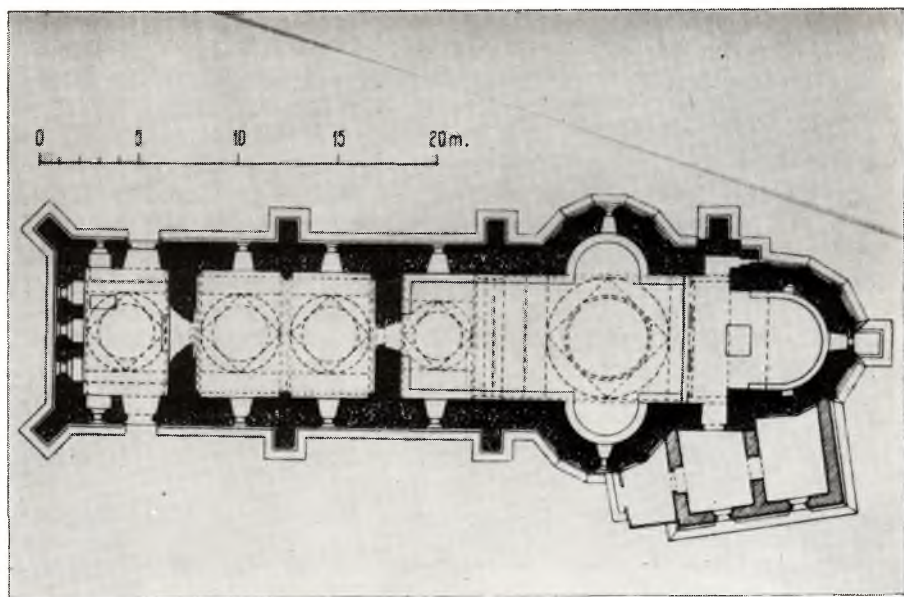
Biserica Înălțarea Domnului — plan.
