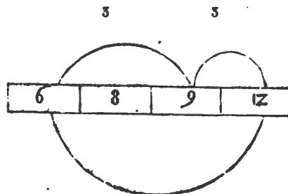
Proportionalitas arithmetica. Differentiæ æquales.
