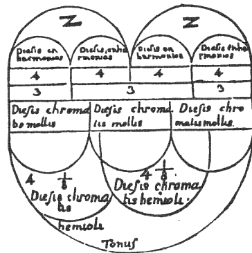
Omnium intervallorum quæ in tono sunt secundum Aristoxenum divisio.
