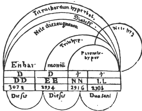
Tetrachordos hyperboleon. Nete hyperboleon. Nete hyperboleon. Nete hyperboleon.
