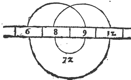
Proportionalitas geometrica. Sesquialteræ proportiones.
