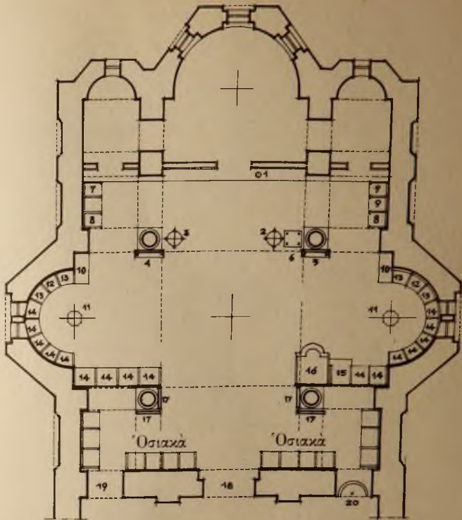
ΣΧ. Α΄ ΚΥΡΙΩΣ ΝΑΟΣ - ΔΑΠΕΔΟΝ
