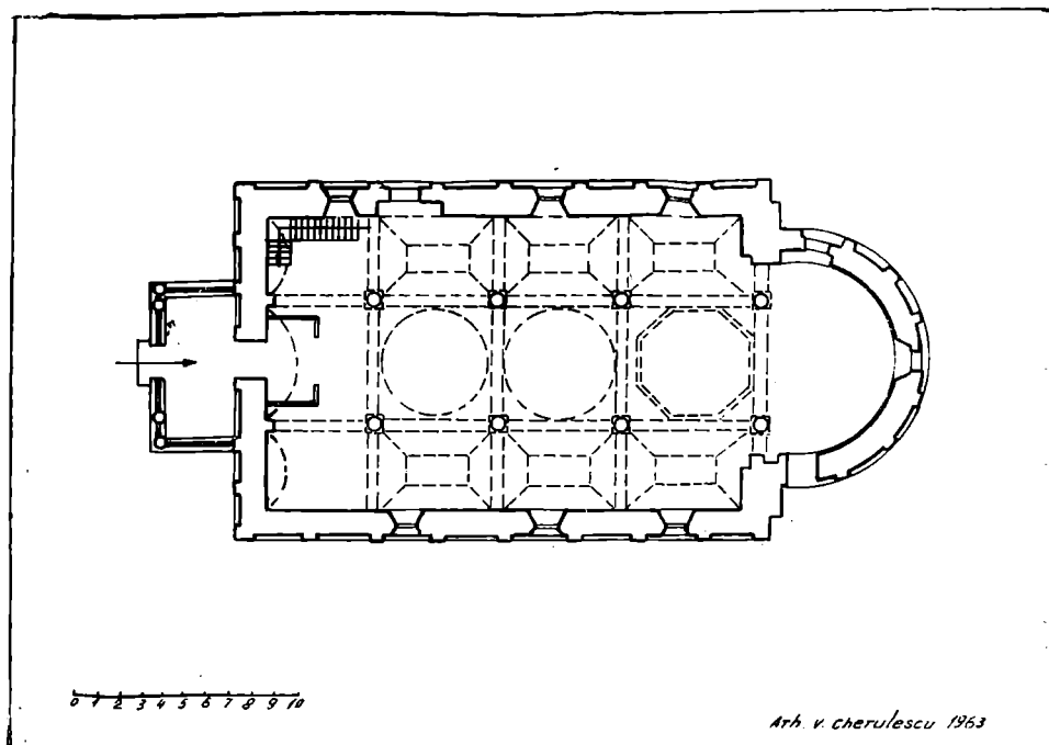
Fig. 2. — Planul bisericii Neguțători din Buzău.
