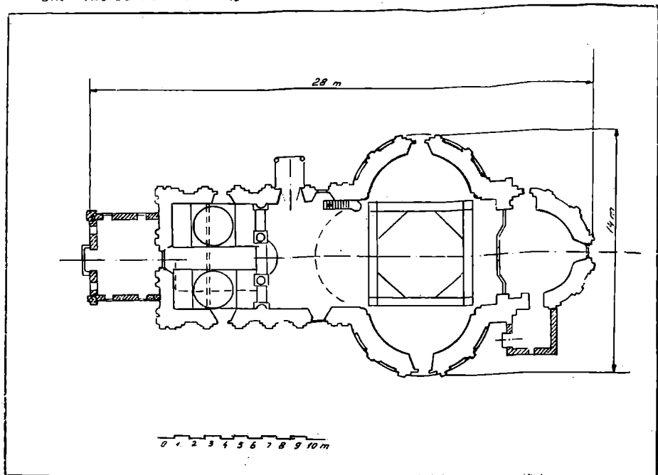
Fig. 7. — Planul bisericii Sfinții Ingeri din Buzău
