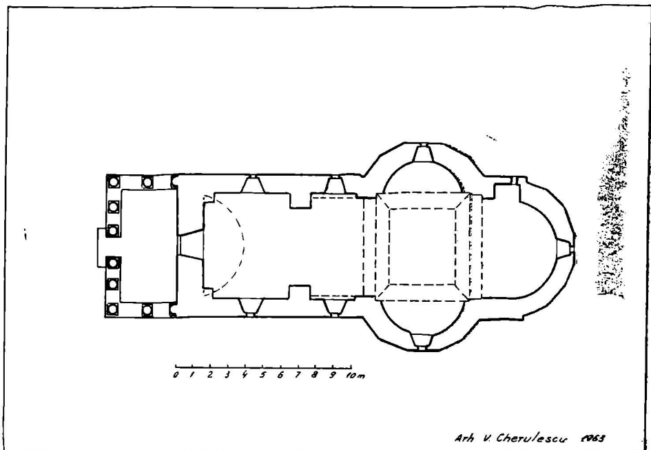
Fig. 5. — Planul bisericii Minăstirii Banu din Buzău
