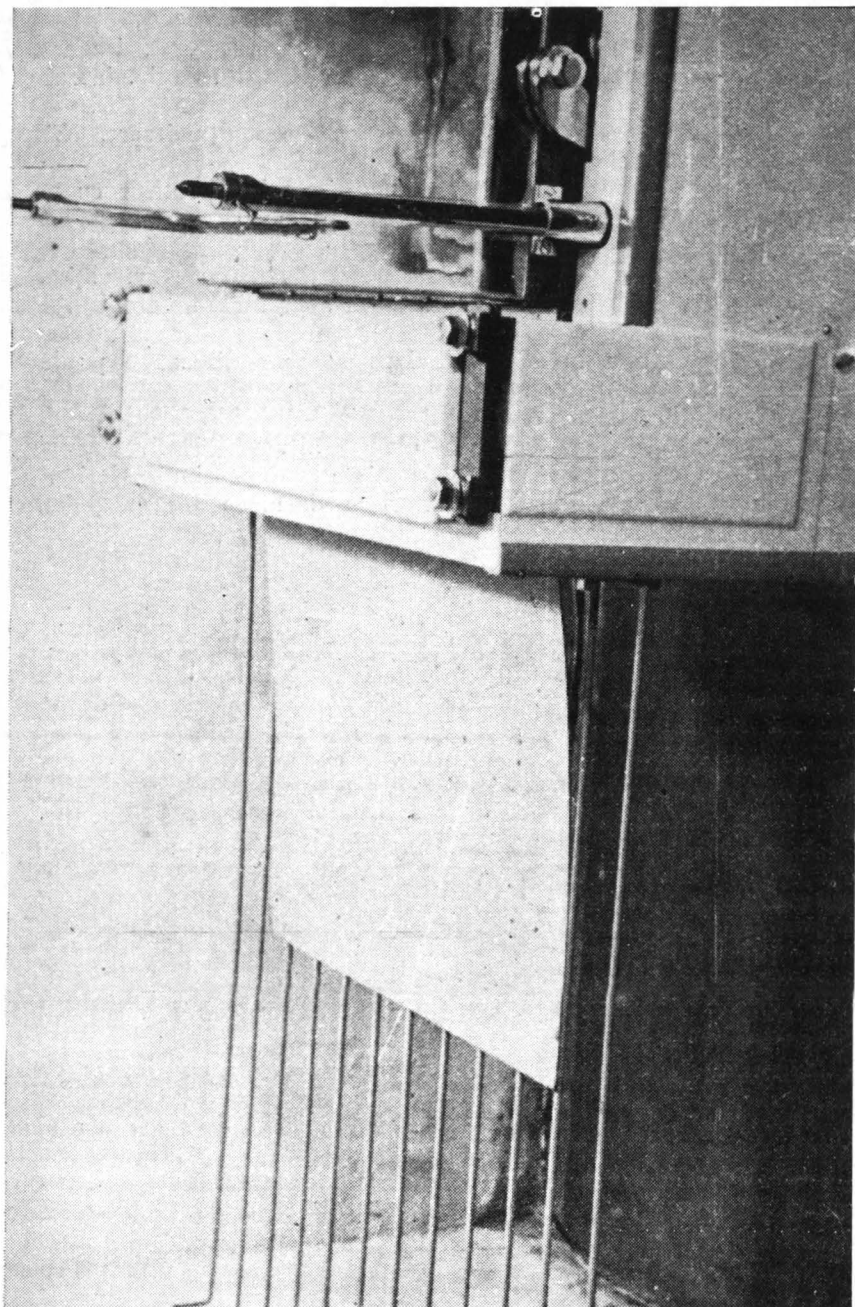
Aparatul de laminat în timpul funcționării. Ieșirea „sandwichului” după laminare.
