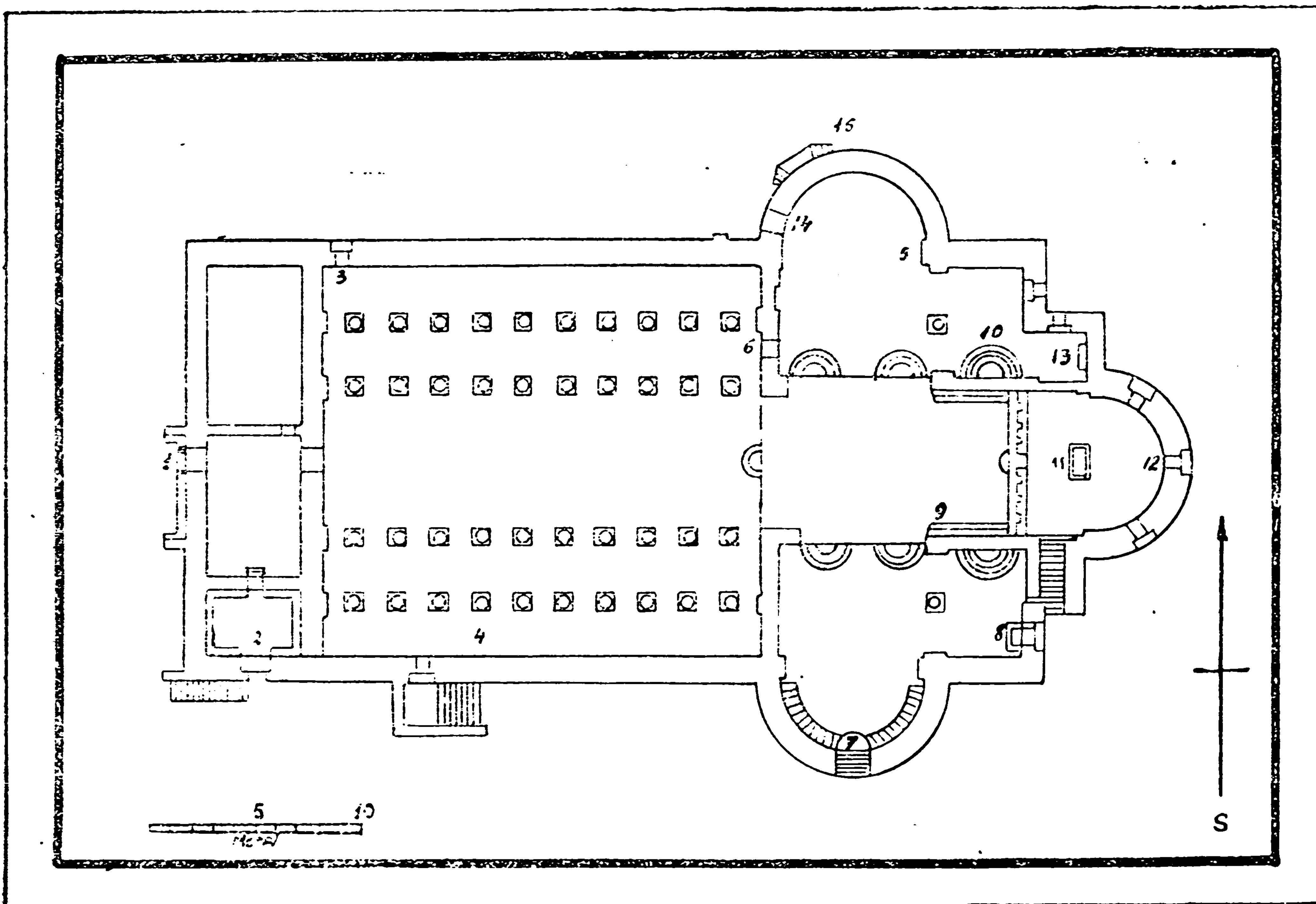
Biserica Nașterii (planul).
