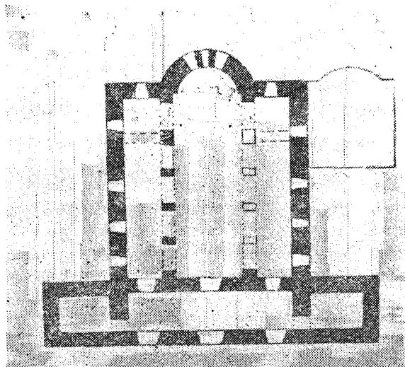
Fig. 5. — Planul bisericii nr. 2, Bir-Bir-Kilissé (După Strzygowski, Kleinasiën ; apud Charles Diehl, op. cit. , fig. 35, p. 97).
