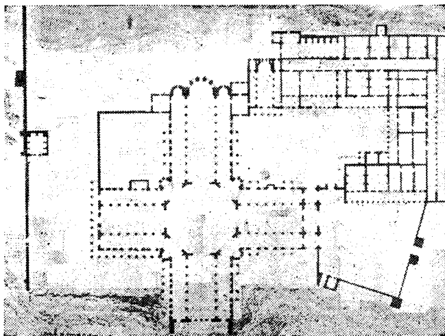
Fig. 16. Planul minăstirii Sfintul Simion Stilitul (După Vögüé, Syrie centrale ; apud Charles Diehl, Manuel d'art byzantin , t. I, Paris, 1925, fig. 6, p. 36).
