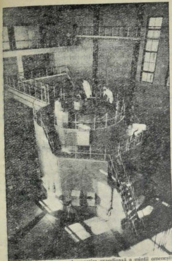
Energia atomică este o descoperire grandioasă a minții omenești. În țara noastră fizica nucleară a luat o mare dezvoltare în ultimii ani, fiind pusă în slujba fericii omului. (În fotografie: reactorul atomic construit cu ajutorul Uniunii Sovietice.)
