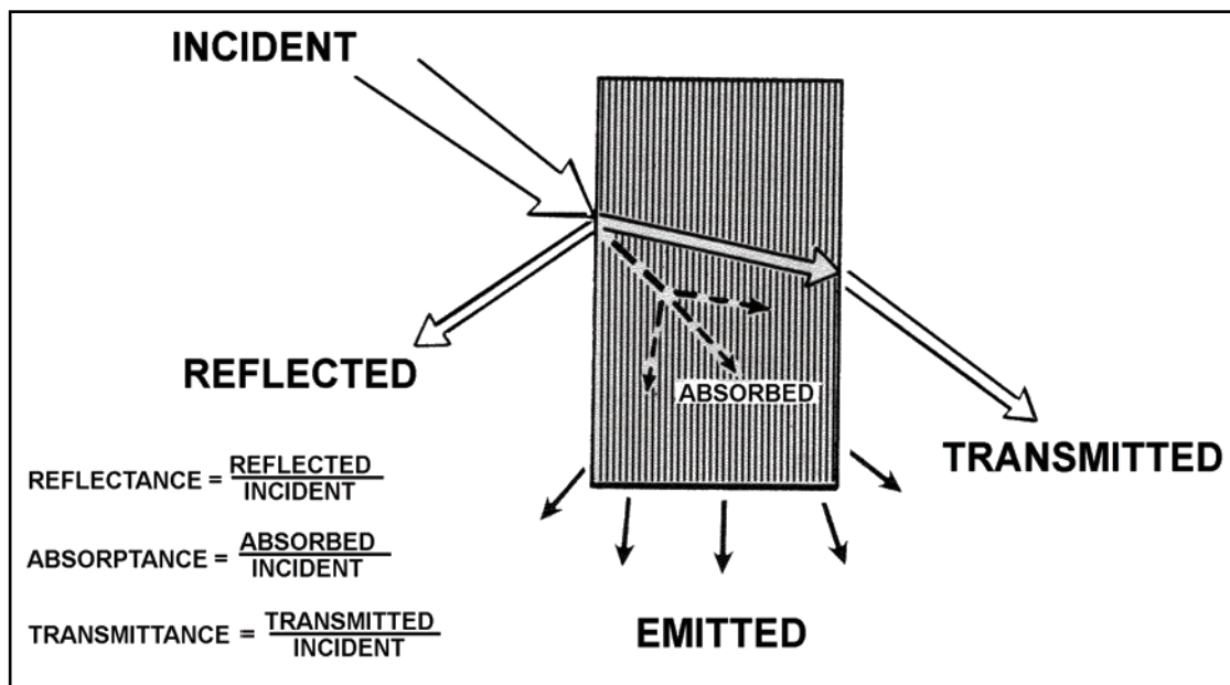
Figure 4-6. IR energy
