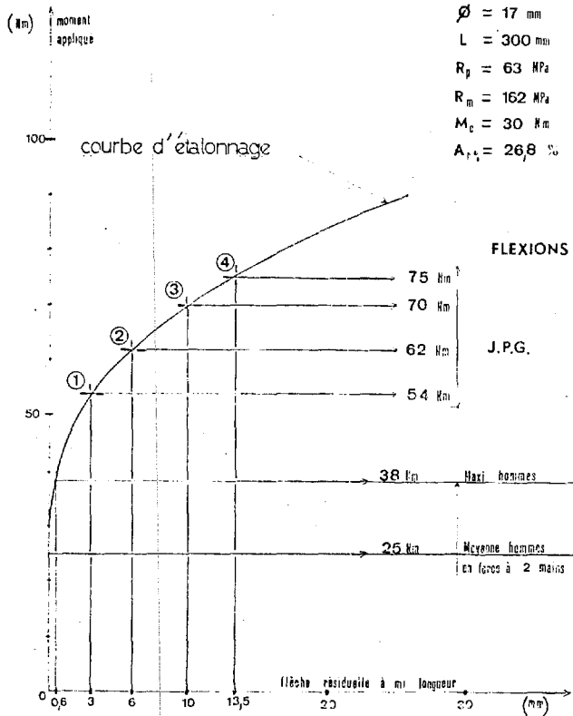
Figure 2. — Diagramme donnant la flèche en fonction du moment appliqué pour une barre témoin identique à celle de la figure 1.
