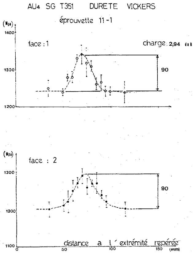
Figure 7. — Duretés mesurées sur les deux faces de l'éprouvette d'alliage léger 11-1, après essai.
