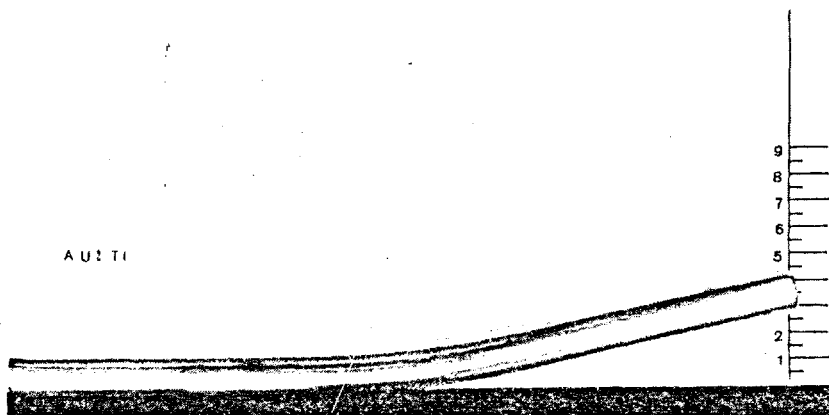
Figure 1. — Photographie de la barre en AU2 de 17 mm de diamètre, après flexion.
