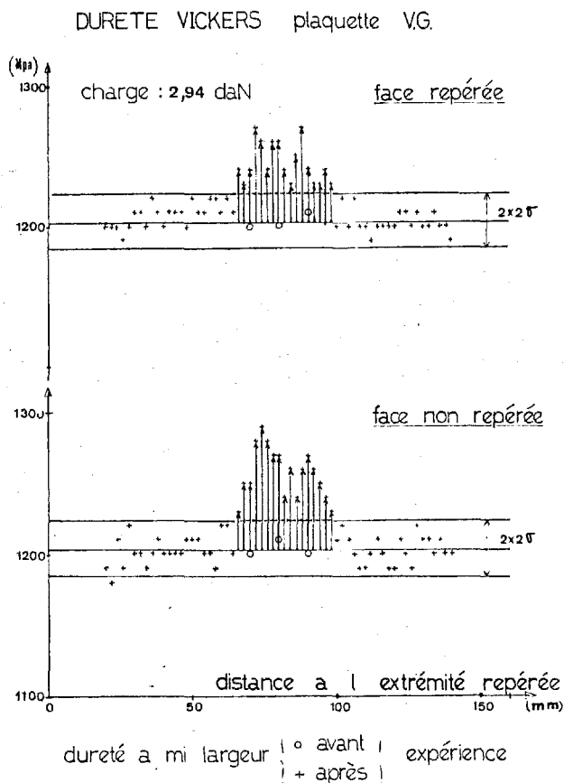
Figure 8. — Dureté mesurée sur les deux faces de l'éprouvette d'alliage léger VG, avant et après essai.
