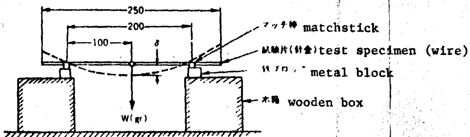
(第1図) 実験装置概略図
