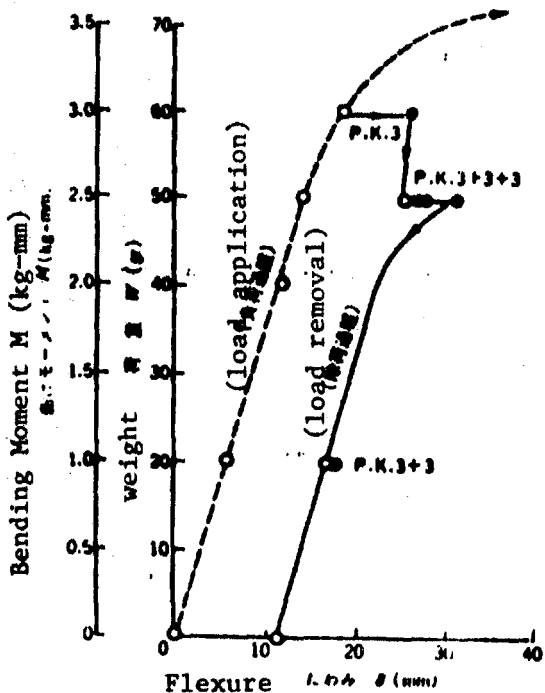
(第4圖) 實驗結果, 例2: 荷重 (曲げモーメント) - たわみ曲線
