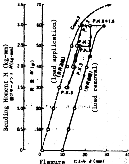
(第5圖) 實驗結果, 例3: 荷重 (曲げモーメント) - たわみ曲線
