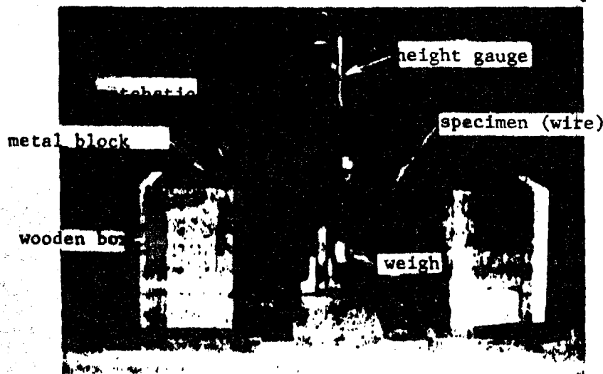
(写真1) 実験装置
