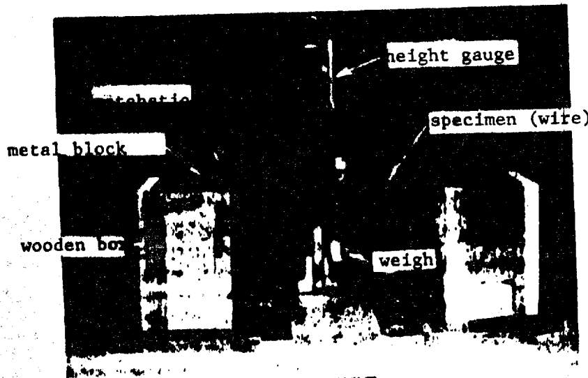
(写真1) 実験装置
