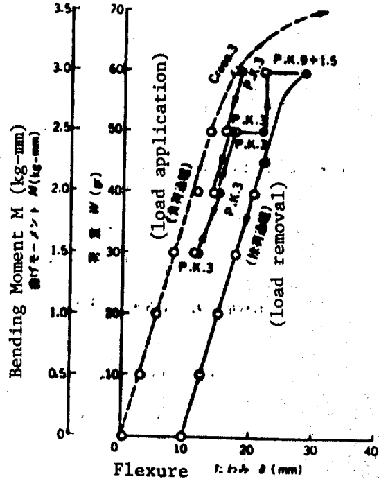
(第5図) 実験結果, 例3: 荷重 (曲げモーメント) - たわみ曲線
