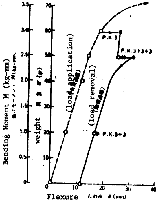
(第4図) 実験結果, 例2: 荷重 (曲げモーメント) - たわみ曲線
