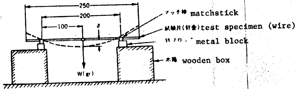
(第1図) 実験装置概略図
